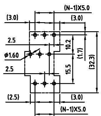
P.C.B. LAYOUT
