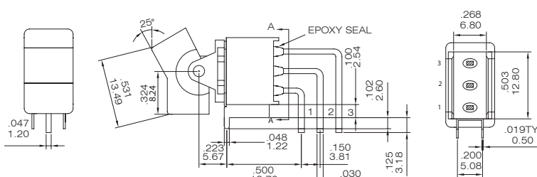
NER8013L- R11-2-Q
