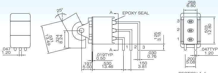
NER8015L- R11-2-Q
