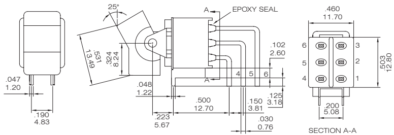
NER8011L- R11-2-Q
