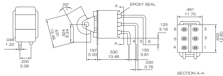
NER8017L- R11-2-Q
