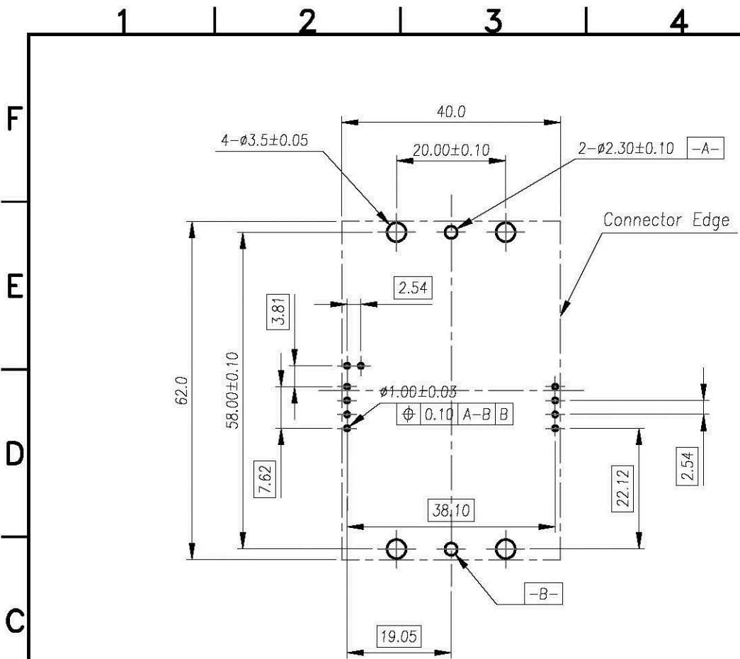
P.C.B. Layout
