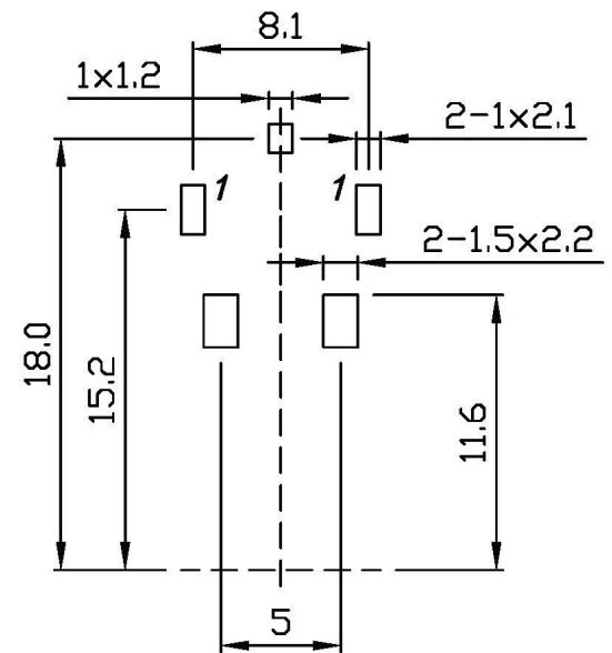
P.C.B LAYOUT(±0.1) (BOTTOM VIEW)
