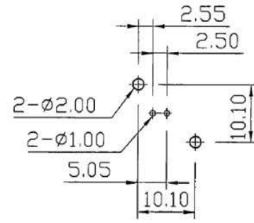
(1 : 1) P.C.B. LAYOUT (印刷电路板配置)
