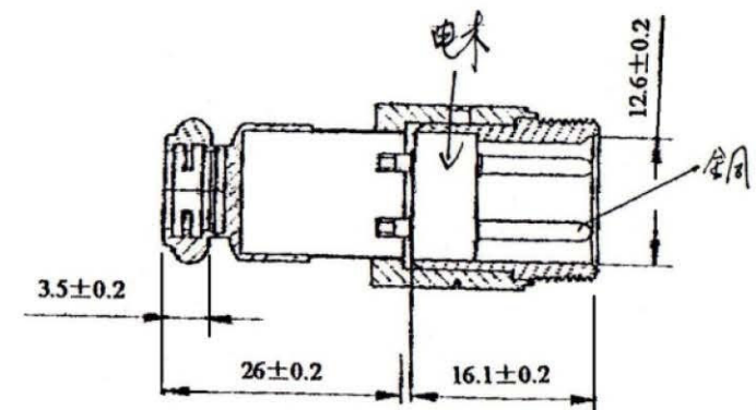
A-A SECTION
