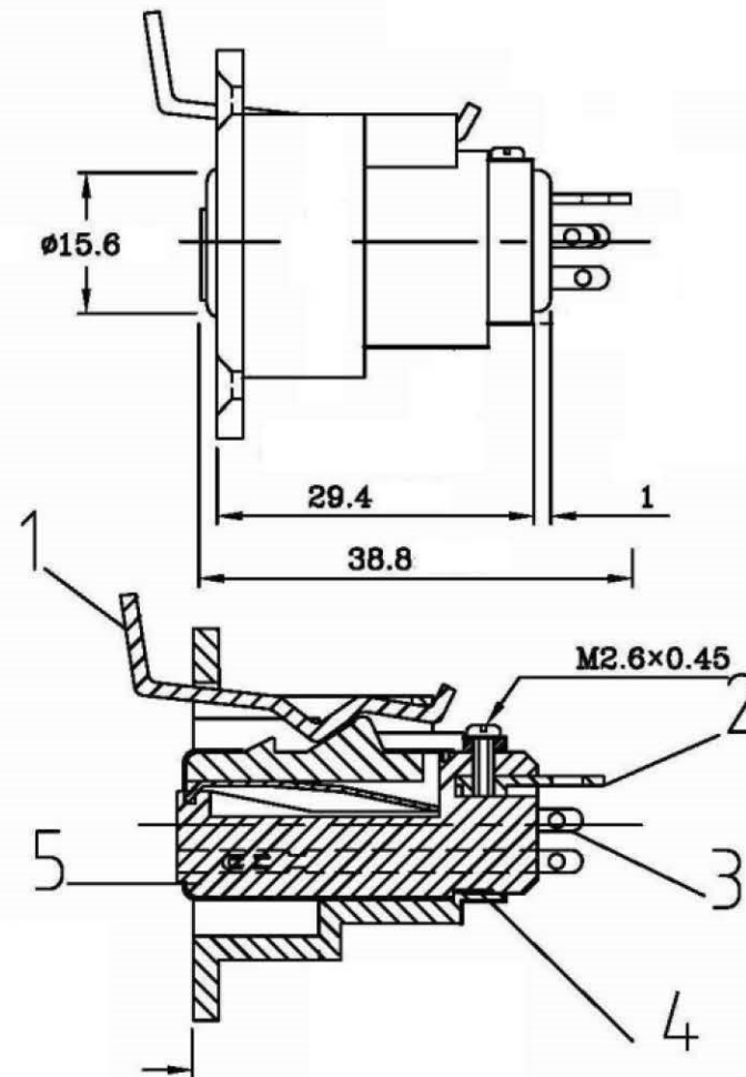
A-A SECTION
