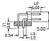
R1 TYPE
