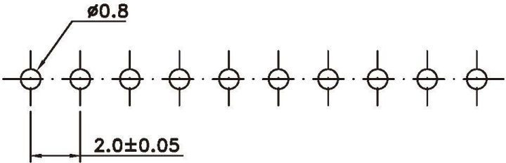
P.C.B. LAYOUT
