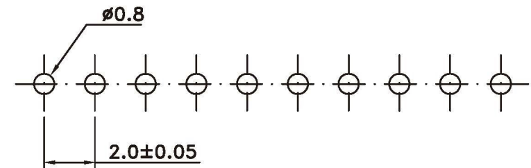
P.C.B. LAYOUT
