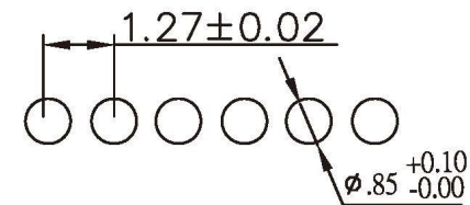
P.C.Board Layout
