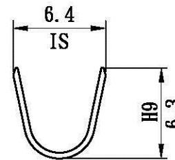
A-A Section
