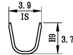
A-A Section
