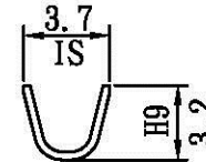
A-A Section
