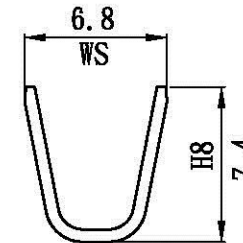
A-A Section
