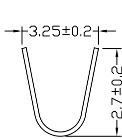
A-A SEC
