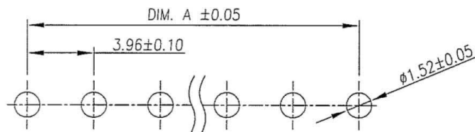
P.C.B LAYOUT
