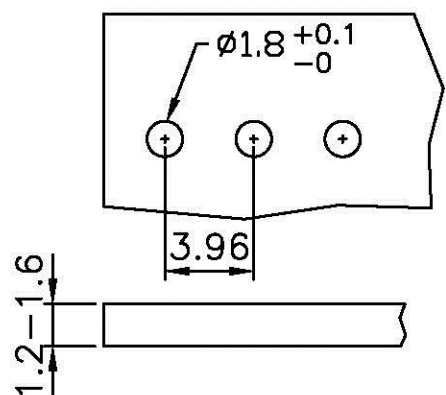
P.C.BOARD LAYOUT
