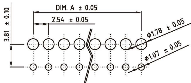
P.C.B LAYOUT
