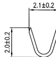
A-A SECTION
