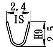
A-A Section
