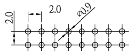
P.C.Board Layout
