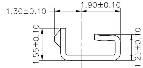
SEC:D-D
