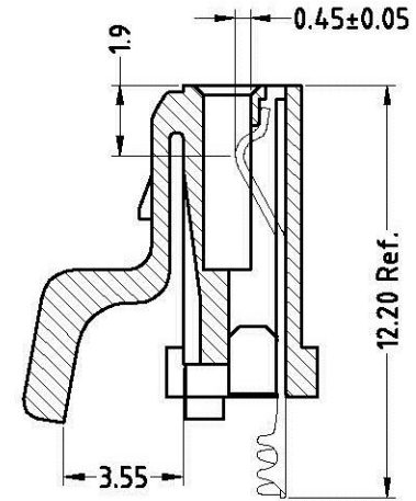
SEC:A-A
