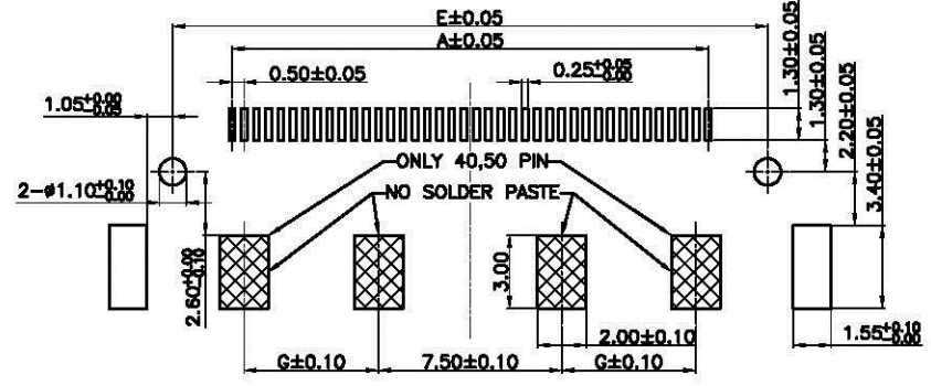
P.C.B. Layout
