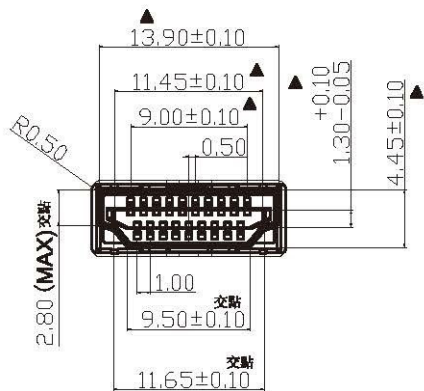
DETAIL A 10:1
