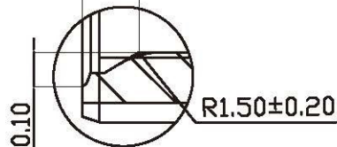
DETAIL A 10:1
