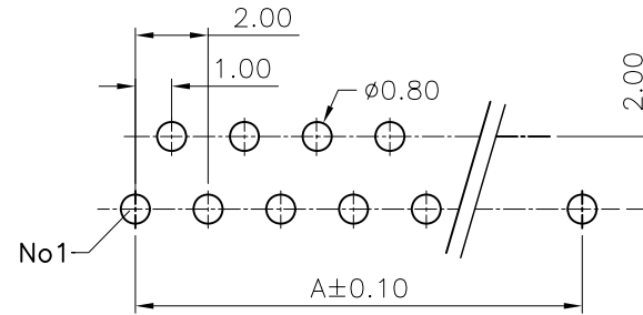
P.C.Board Layout
