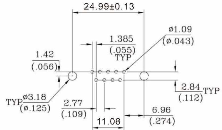
P.C.B LAYOUT
