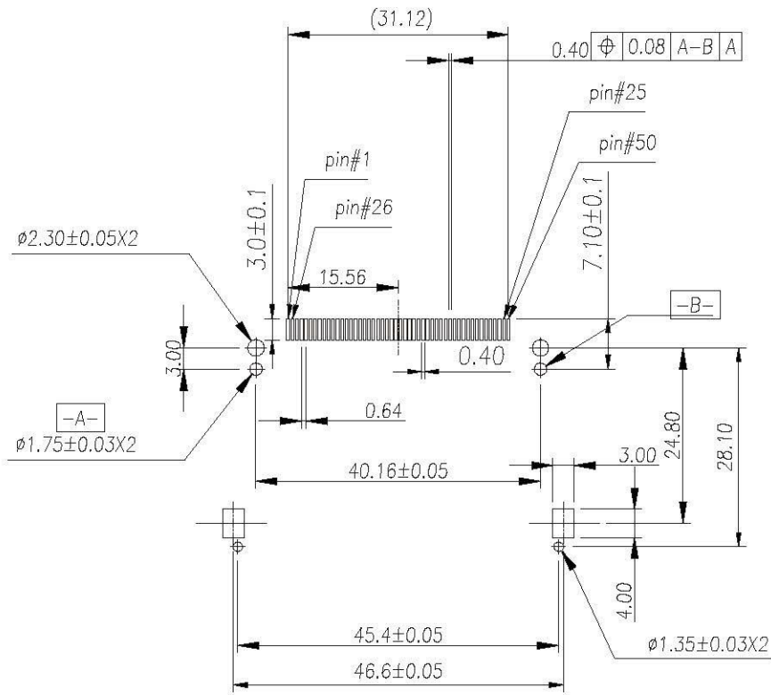
P.C.B Layout
