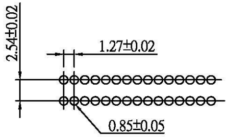
P.C.Board Layout
