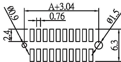
P.C.Board Layout
