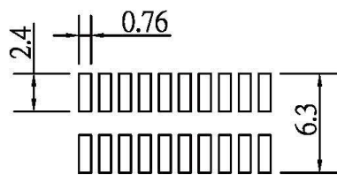
P.C.Board Layout
